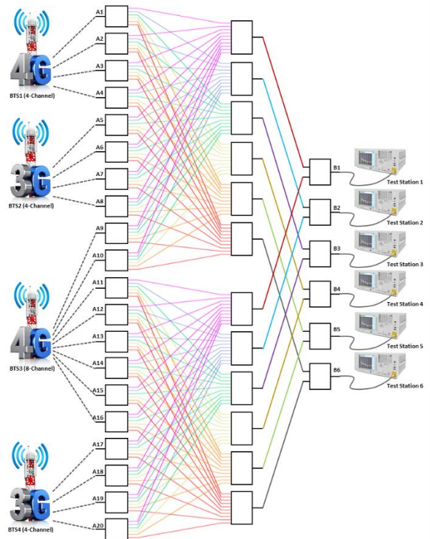
図 2: ZT-20X6NB スイッチマトリックスを利用したマルチユーザベースステーション試験システムの機能図。6 つの独立したテストステーションは 20 BTS チャンネルはすべて相互接続できる。
