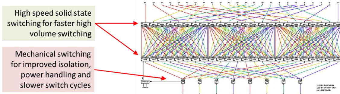
図 4. 各々のスイッチの特長を生かした最適設計スイッチマトリックス
